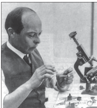
Уладзіслаў Старэвіч
